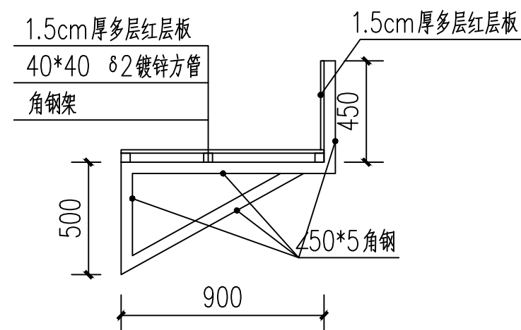
∠50×5角钢支撑架侧立面图
