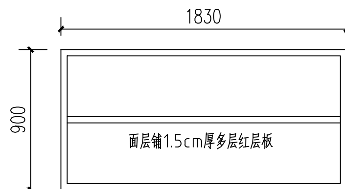
40×40 82镀锌方管 平面图
