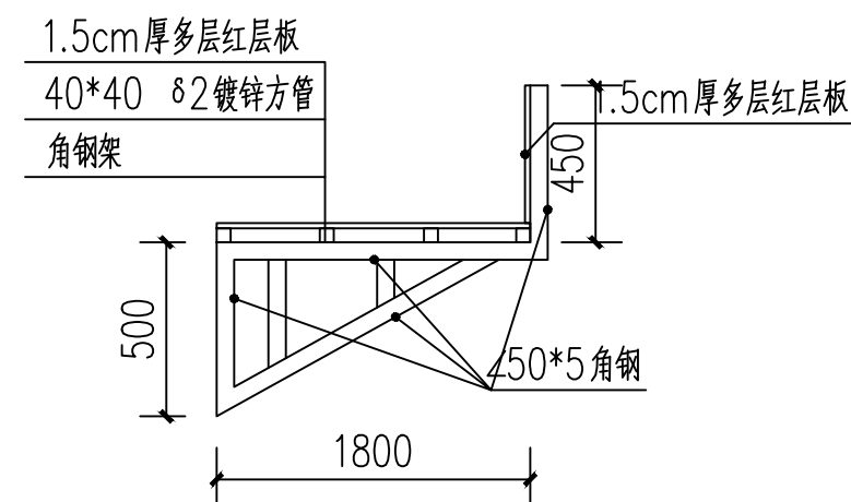
∠50×5角钢支撑架侧立面图
